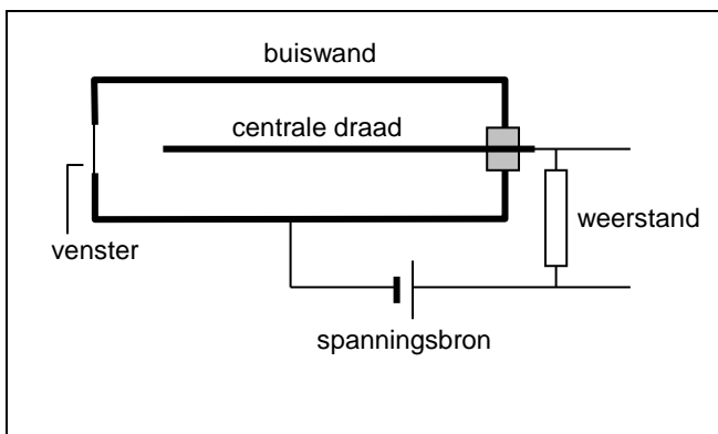
Figuur 1 – De GM-telbuis.
