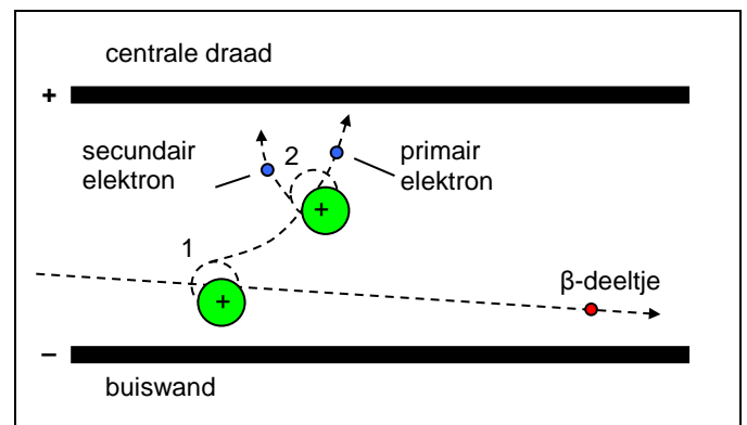
Figuur 2 – Het lawine-effect in de GM-telbuis.
